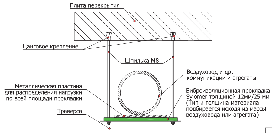
6.4 Схема закрепления труб, воздуховодов и др. коммуникаций и агрегатов к перекрытию при помощи траверсы и виброизоляционного материала Sylomer
