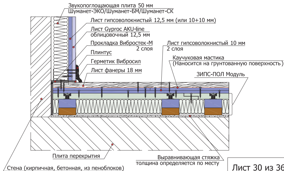
5.6.8 Схема примыкания конструкции ЗИПС-ПОЛ Модуль к каркасной облицовке
