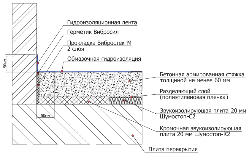
5.8.3 Схема устройства гидроизоляции в конструкции плавающего пола с применением звукоизолирующих плит Шумостоп в один слой
