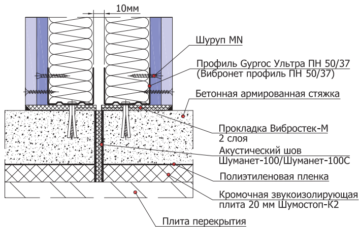
Примыкание перегородки на двойном 2x50 мм (независимом) каркасе к конструкции "плавающего" пола
