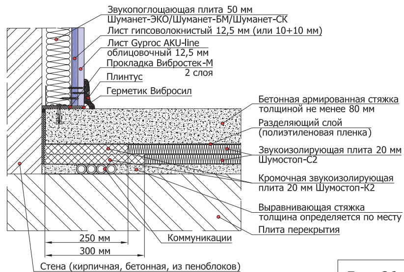
5.4.8 Схема примыкания конструкции плавающего пола с применением звукоизолирующих плит Шумостоп в два слоя к стене и коммуникациями под стяжкой
