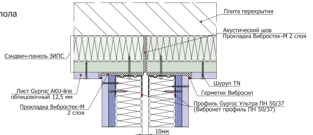
Примыкание перегородки на двойном 2x50 мм (независимом) каркасе к панелям ЗИПС на потолочном перекрытии
