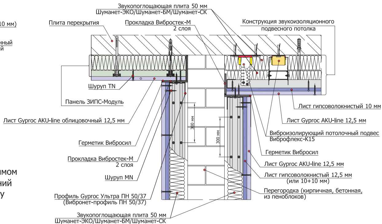
3.2.2 Примыкание облицовки стены на независимом сдвоенном каркасе 50 мм к панелям ЗИПС на потолочном перекрытии и подвесному звукоизолирующему потолку
