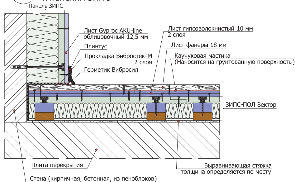
5.6.6 Схема примыкания конструкции ЗИПС-ПОЛ Модуль к панелям ЗИПС
