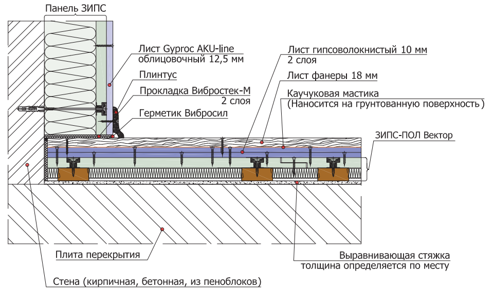
5.6.2 Схема примыкания конструкции ЗИПС-ПОЛ Вектор к панелям ЗИПС
