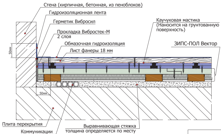
5.8.4 Схема устройства гидроизоляции в конструкции пола с применением панелей ЗИПС-ПОЛ
