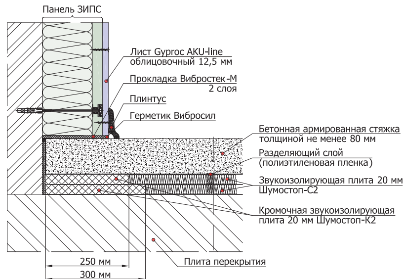
5.4.8 Схема примыкания конструкции плавающего пола с применением звукоизолирующих плит Шумостоп в два слоя к стене и коммуникациями под стяжкой
