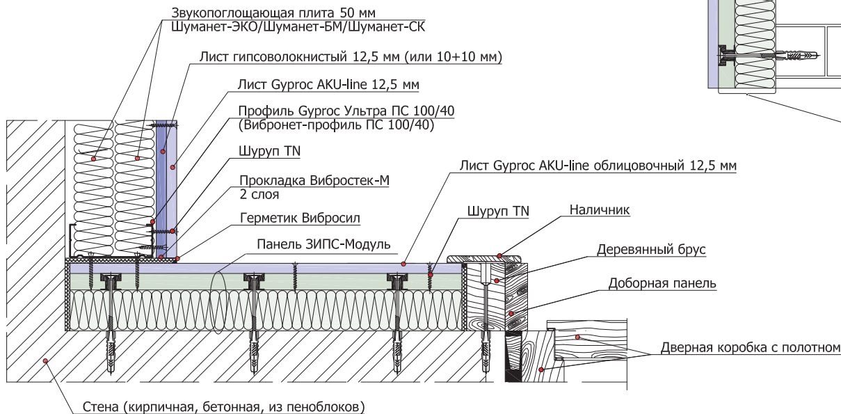
2.3.3 Угловое примыкание панелей ЗИПС-Модуль на стене к облицовке на каркасе 100 мм и дверному проему
