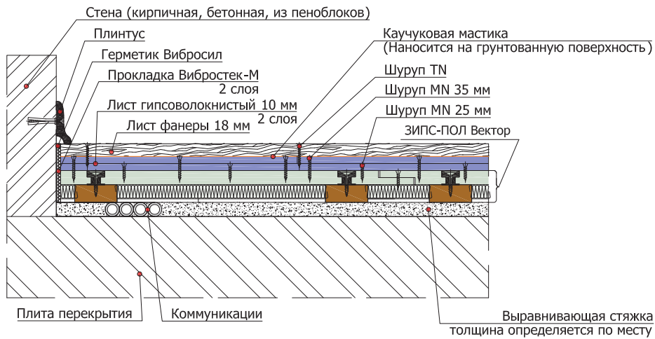
5.6.1 Схема устройства конструкции ЗИПС-ПОЛ Вектор
