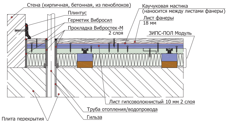
5.6.7 Схема примыкания конструкции ЗИПС-ПОЛ Модуль к стене и трубе отопления/водопровода (монтаж на ровное перекрытие)
