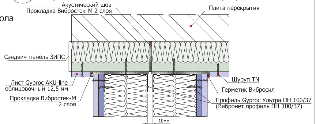
1.3.4 Примыкание перегородки на двойном 2x100 мм (независимом) каркасе к панелям ЗИПС на потолочном перекрытии
