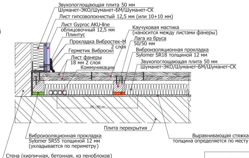
Схема примыкания конструкции пола по деревянным лагам с применением виброизоляционного материала Sylomer к каркасной облицовке
