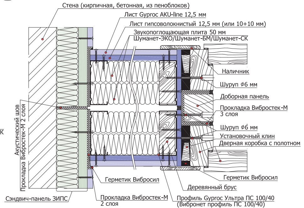
1.3.2 Примыкание перегородки на двойном 2x100 мм (независимом) каркасе к панелям ЗИПС на стене и дверному проему
