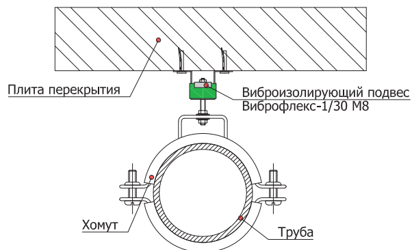
6.3 Схема закрепления труб к потолку при помощи хомута и виброизолирующего крепления Виброфлекс-1/30 М8
