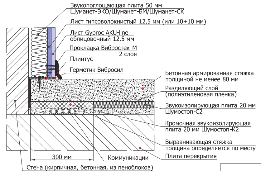
5.4.4 Схема примыкания конструкции плавающего пола с применением звукоизолирующих плит Шумостоп в один слой к стене и коммуникациями под стяжкой
