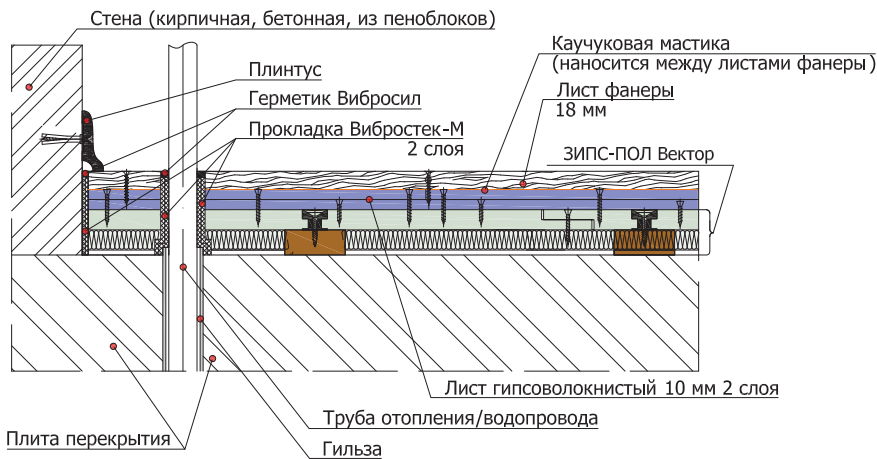
5.6.3 Схема примыкания конструкции ЗИПС-ПОЛ Вектор к стене и трубе отопления/водопровода (монтаж на ровное перекрытие)
