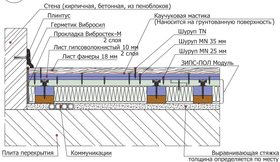
5.6.5 Схема устройства конструкции ЗИПС-ПОЛ Модуль
