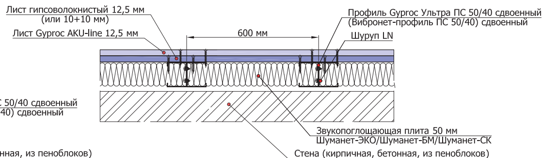
3.2.4 Облицовка стены на независимом сдвоенном каркасе 50 мм горизонтальный разрез
