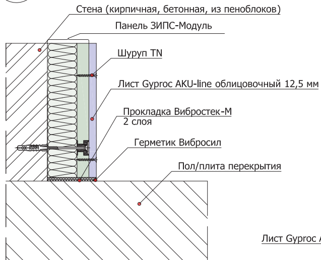
2.3.1 Примыкание панелей ЗИПС-Модуль к перекрытию пола/ потолка
