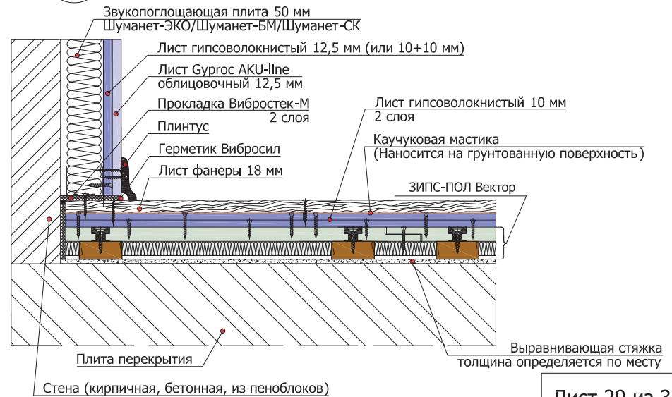
5.6.4 Схема примыкания конструкции ЗИПС-ПОЛ Вектор к каркасной облицовке
