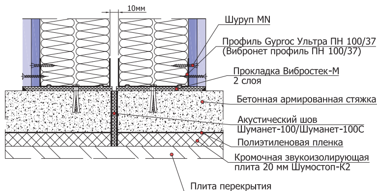
1.3.3 Примыкание перегородки на двойном 2x100 мм (независимом) каркасе к конструкции "плавающего" пола
